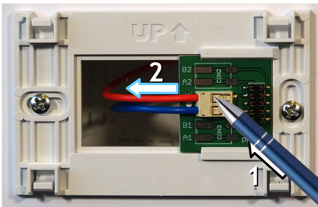
Ilustracja 3: Odłączanie przewodów.
